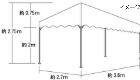
約3坪[約9.5㎡]4本柱
